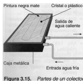
Figura 3.15. Partes de un colector.
